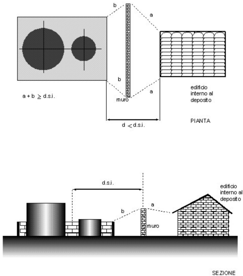
Tavola 7b - Unità di deposito all'aperto: riduzione della distanza di sicurezza interna
