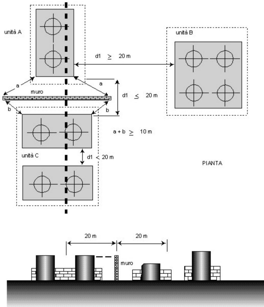
Tavola 3 - Unità di deposito all'aperto
