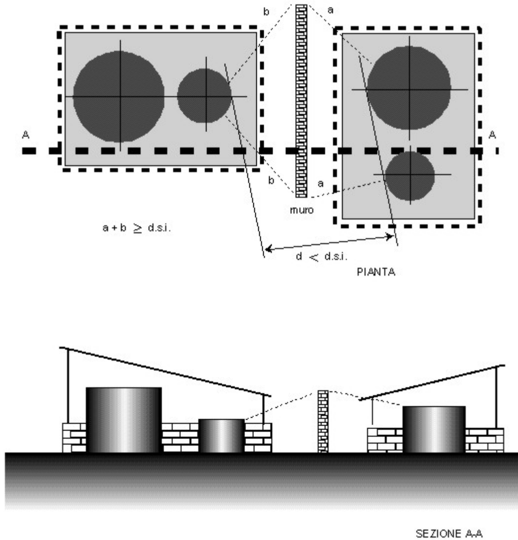
Tavola 4 - Unità di deposito al chiuso: riduzione della distanza di sicurezza interna
