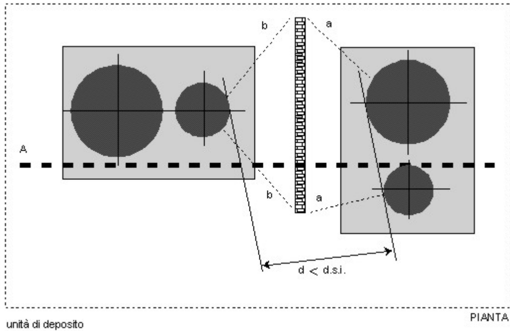
Tavola 7a - Unità di deposito all'aperto: riduzione della distanza di sicurezza interna
