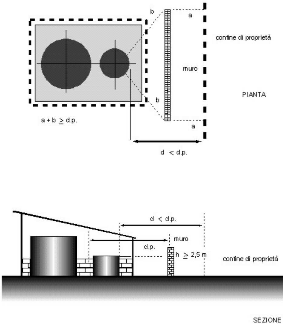
Tavola 5 - Unità di deposito al chiuso: riduzione della distanza di protezione
